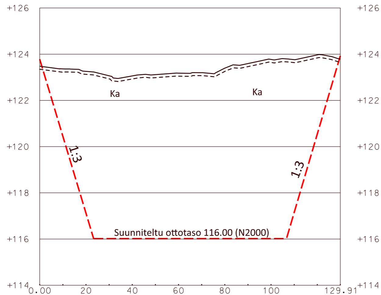
B-B
