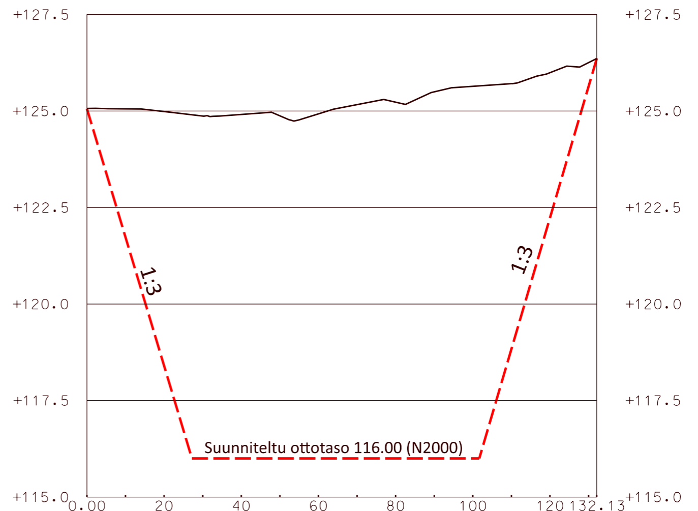
C-C
